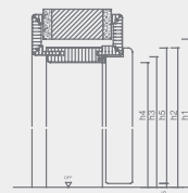
Coupe verticale du revêtement (RF)
