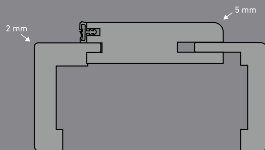
ZARGE MIT RUNDKANTE CHÂSSIS AVEC CHANTS ARRONDIS
