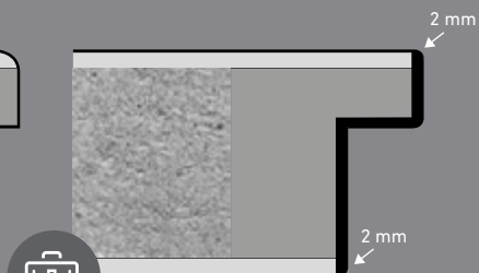
PREMIUMKANTE (PK2) CHANT PREMIUM (PK2)
